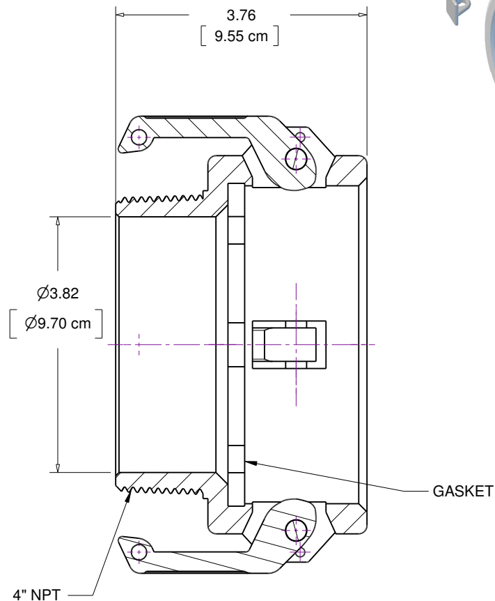
Section A-A
